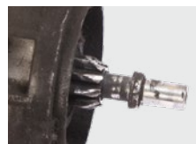
Izglodan pogonski zupčanik
