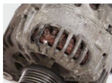
Polomljeno jedno rebro
