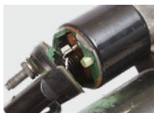
Oštećenje na plastičnom dijelu solenoida
