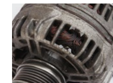
Više od jedno odlomljeno rebro
